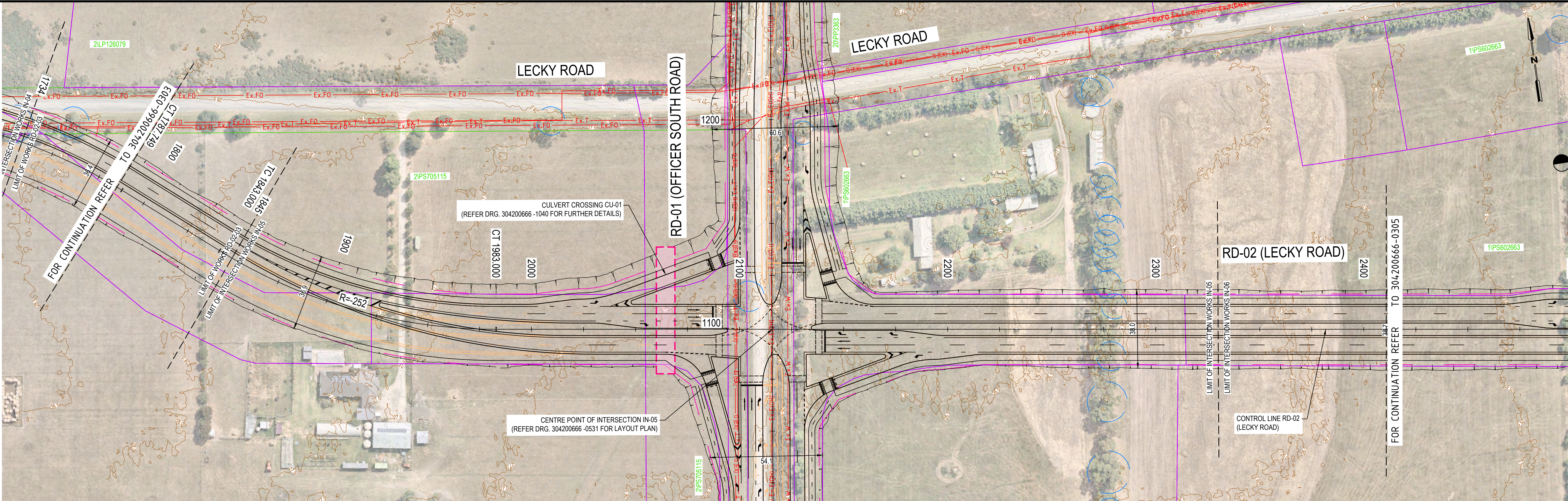
PLAN SCALE: 1:1000
