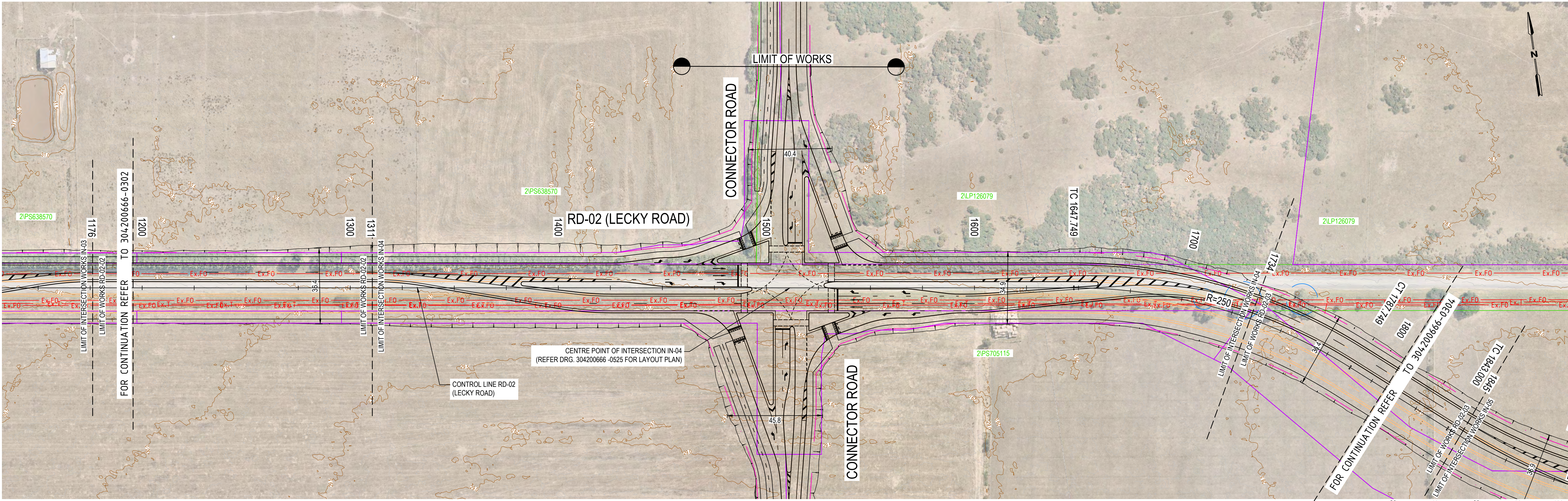
PLAN SCALE: 1:1000
