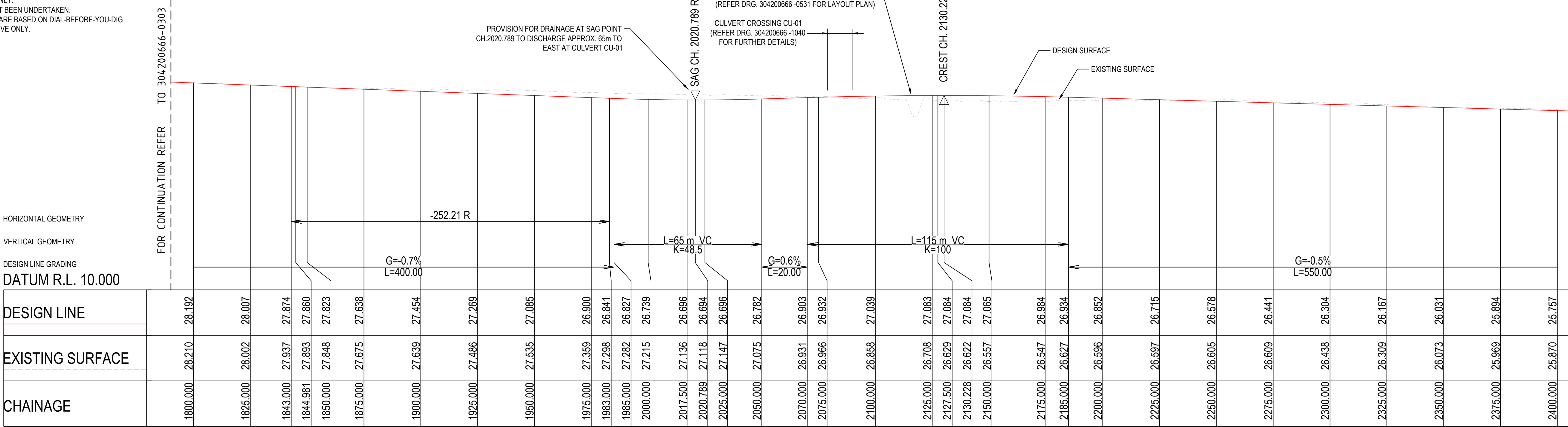
LONGITUDINAL SECTION - RD-02 (LECKY ROAD) SCALE: 1:1000 H 1:200 V
